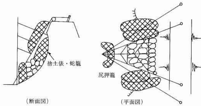
人力設置（作業中ののりくずれに特に注意）
